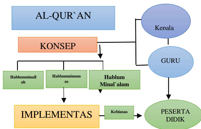
Gambar 1. Kerangka Berpikir
