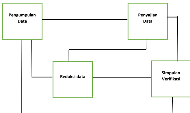
Gambar 2. Analisis
